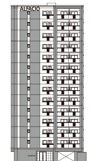
EAST 東側立面図
